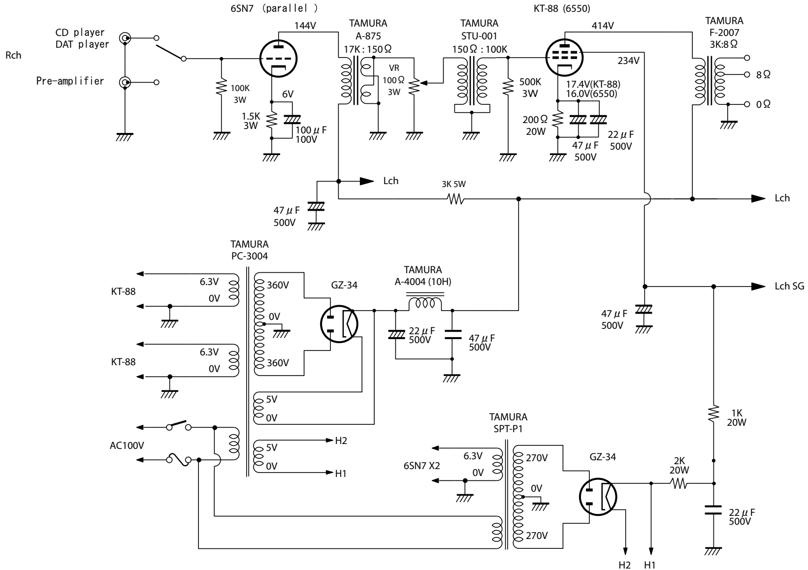
佐久間駿氏設計・製作 KT-88 ステレオパワーアンプ回路図
