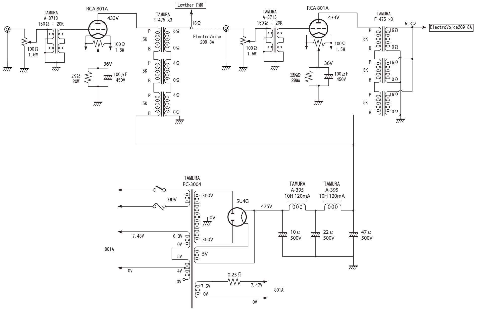
佐久間駿氏制作 801A シングル単段ステレオ・パワーアンプ
