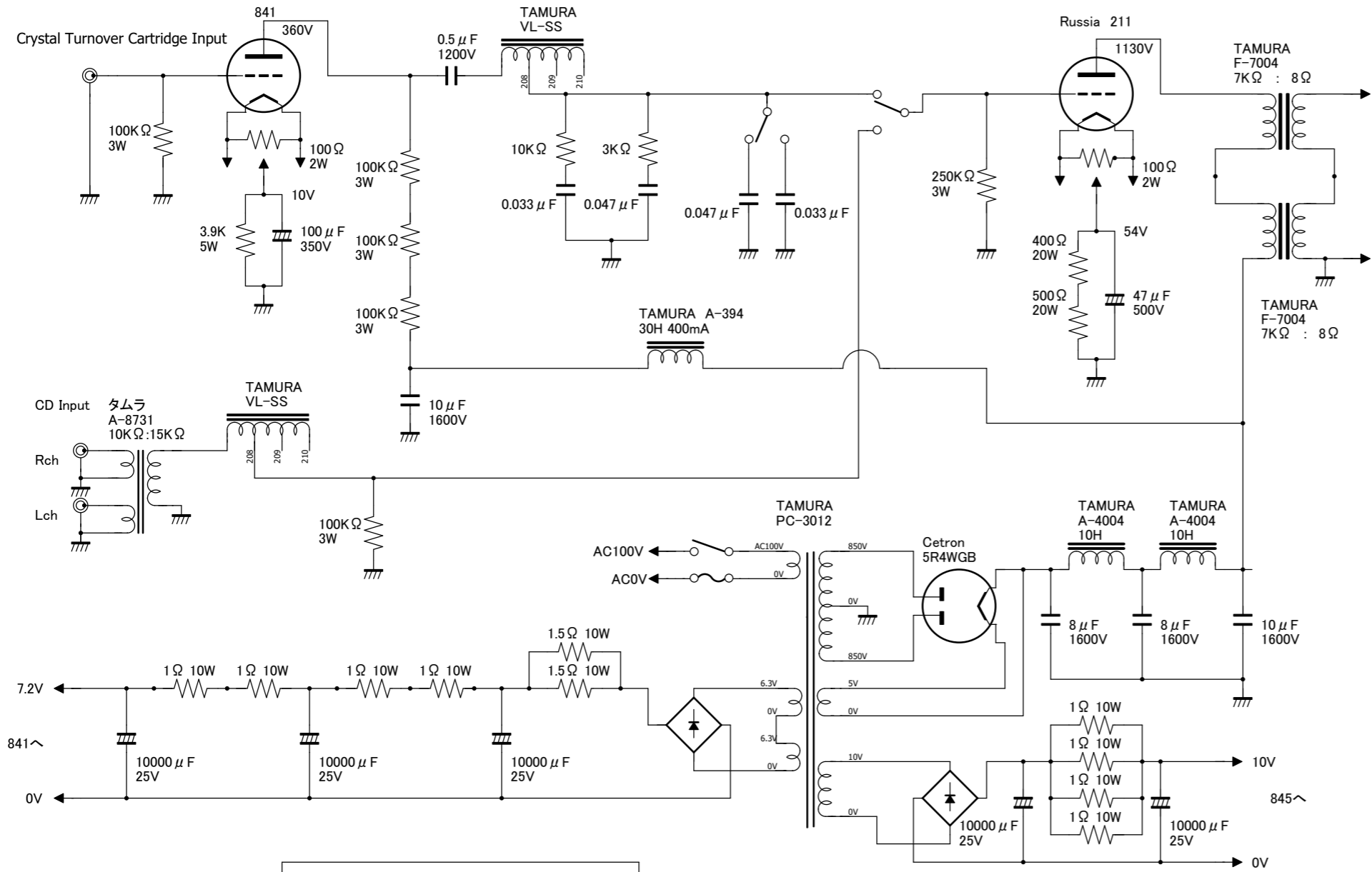
佐久間 駿設計 841と211によるクリスタルカートリッジ用フォノEQアンプ 2017年9月14日
