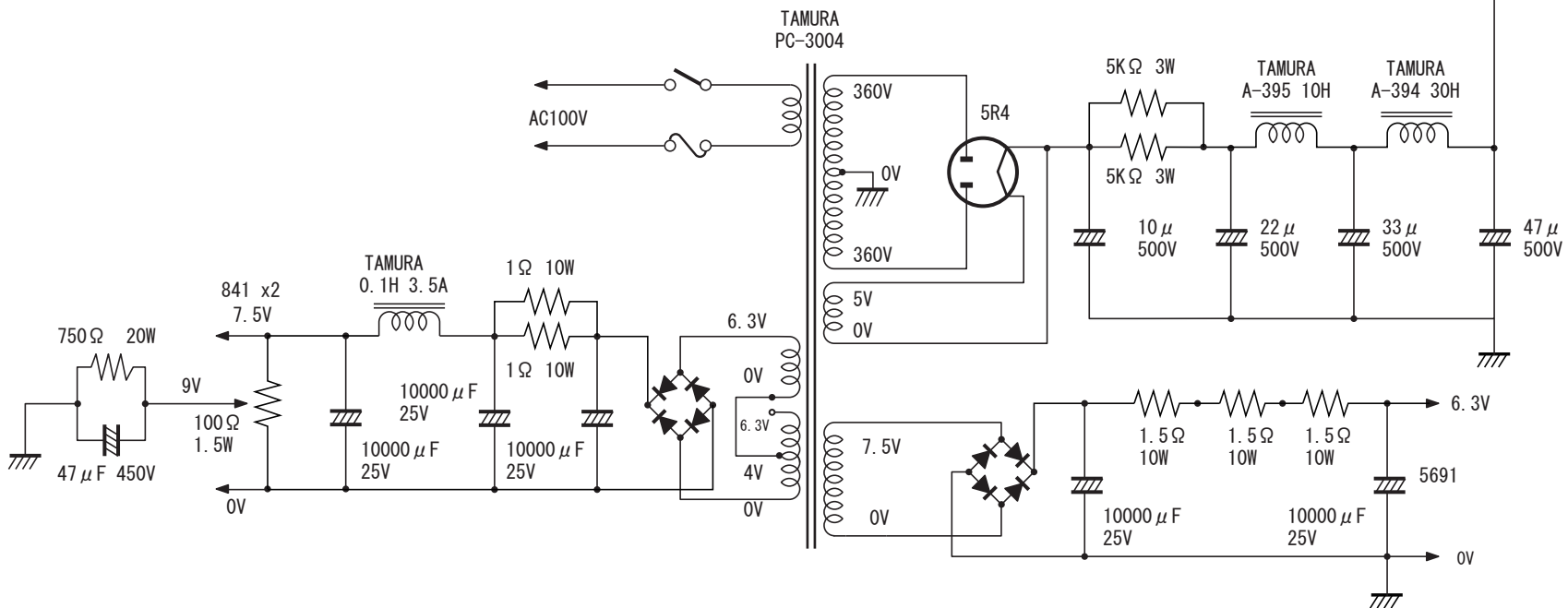
佐久間駿氏製作 841parallelシングル・フォノイコライザーアンプ
